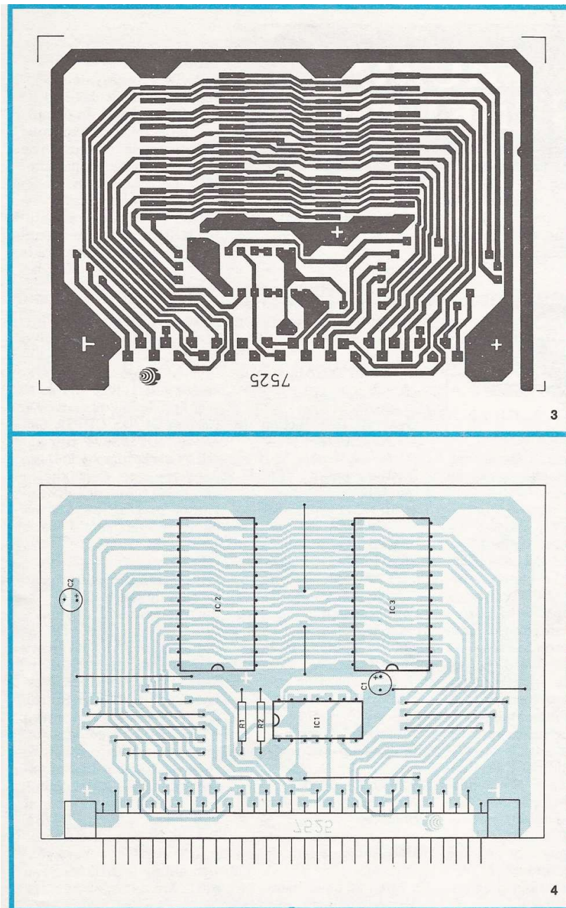
Afb. 3. Printontwerp voor de EPROM-kaart.
