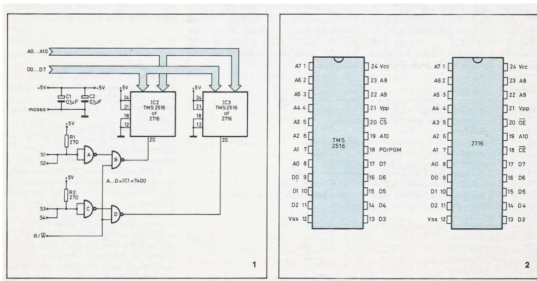
Afb. 1. Schema van de EPROM-kaart voor 4 Kbytes geheugen.
